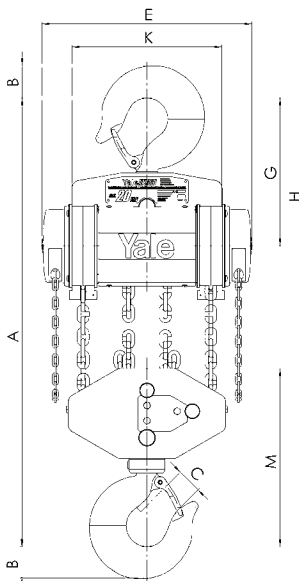
Modell Yalelift 360, 20.000 kg, sechssträngig
