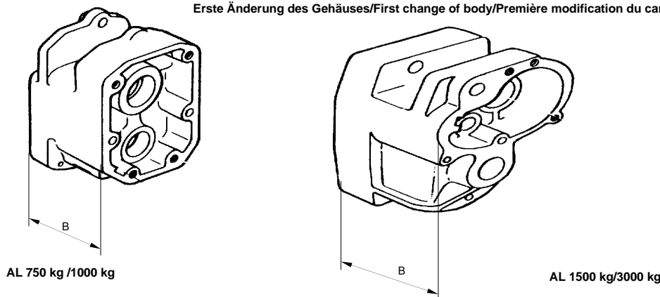
Erste Änderung des Gehäuses/First change of body/Première modification du carter
