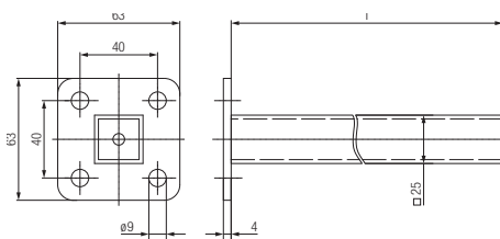
Mitnehmerarm
