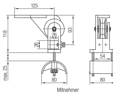
Mitnehmer
