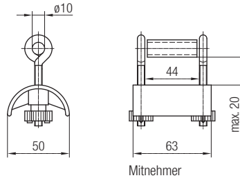
Mitnehmer
