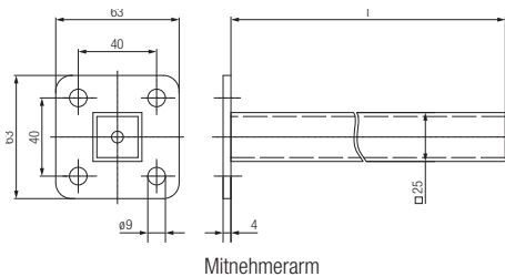
Mitnehmerarm
