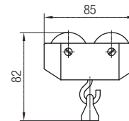
Wagen mit Öse Bestell-Nr. 021116 Tragfähigkeit: 6 kg
